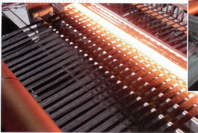
多錘式開織装置 Multi-tow Spreading Machine
